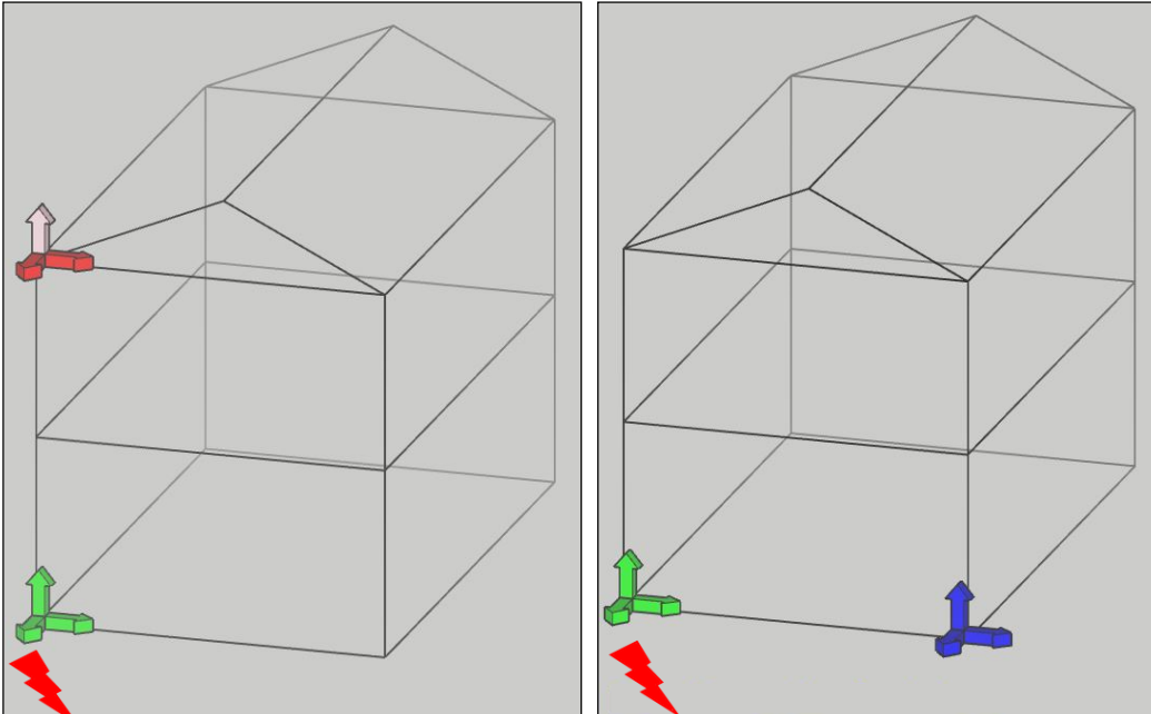
Figuur 8.2 Meetpositie beperkte meting voor de draagconstructie (links) en fundering (rechts) ten opzichte van de bron (rode bliksemschicht).
